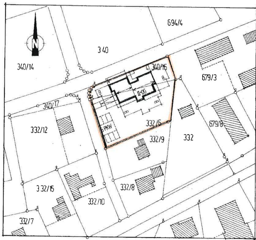
LAGEPLAN M 1:1000
