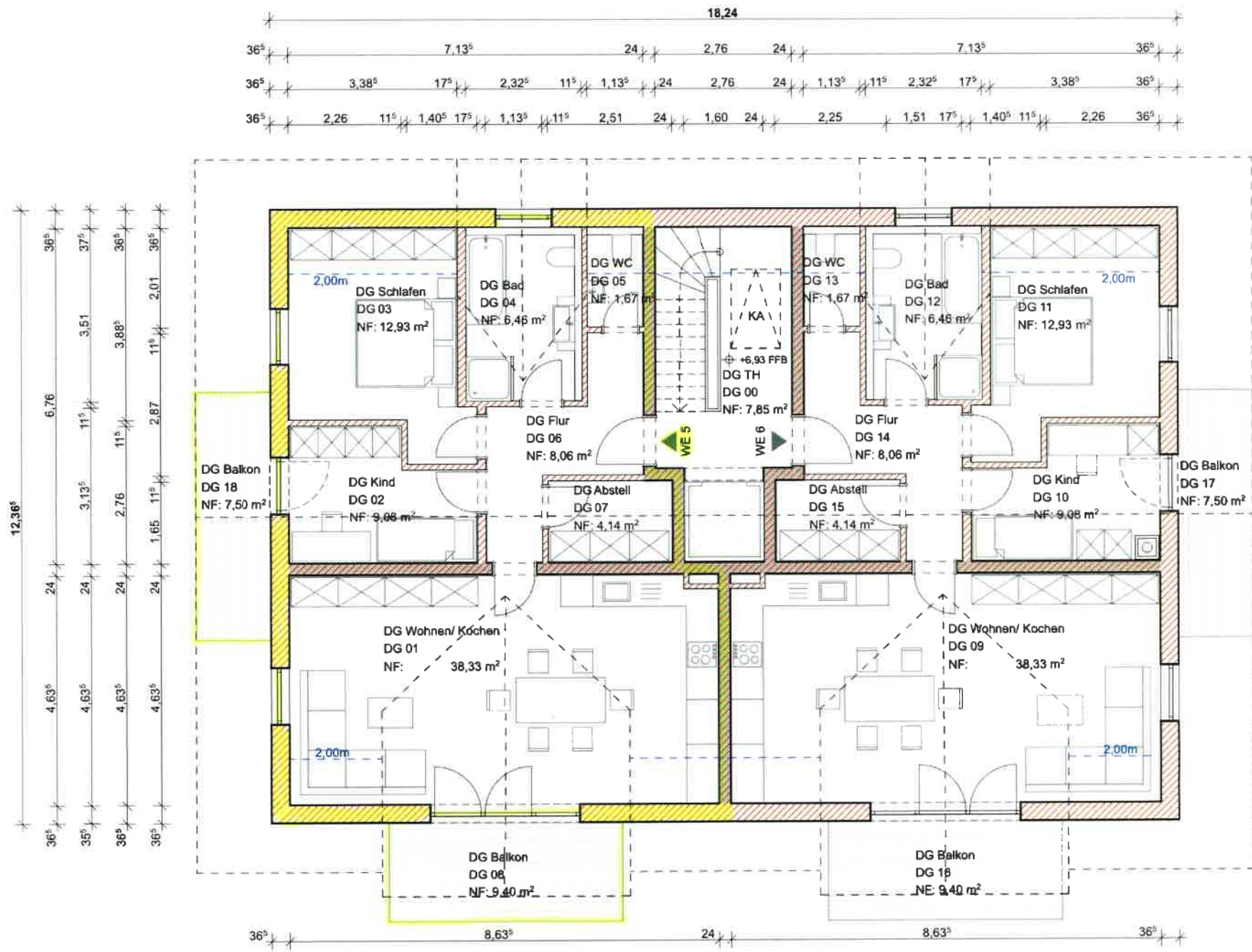
DACHGESCHOß 1:100
