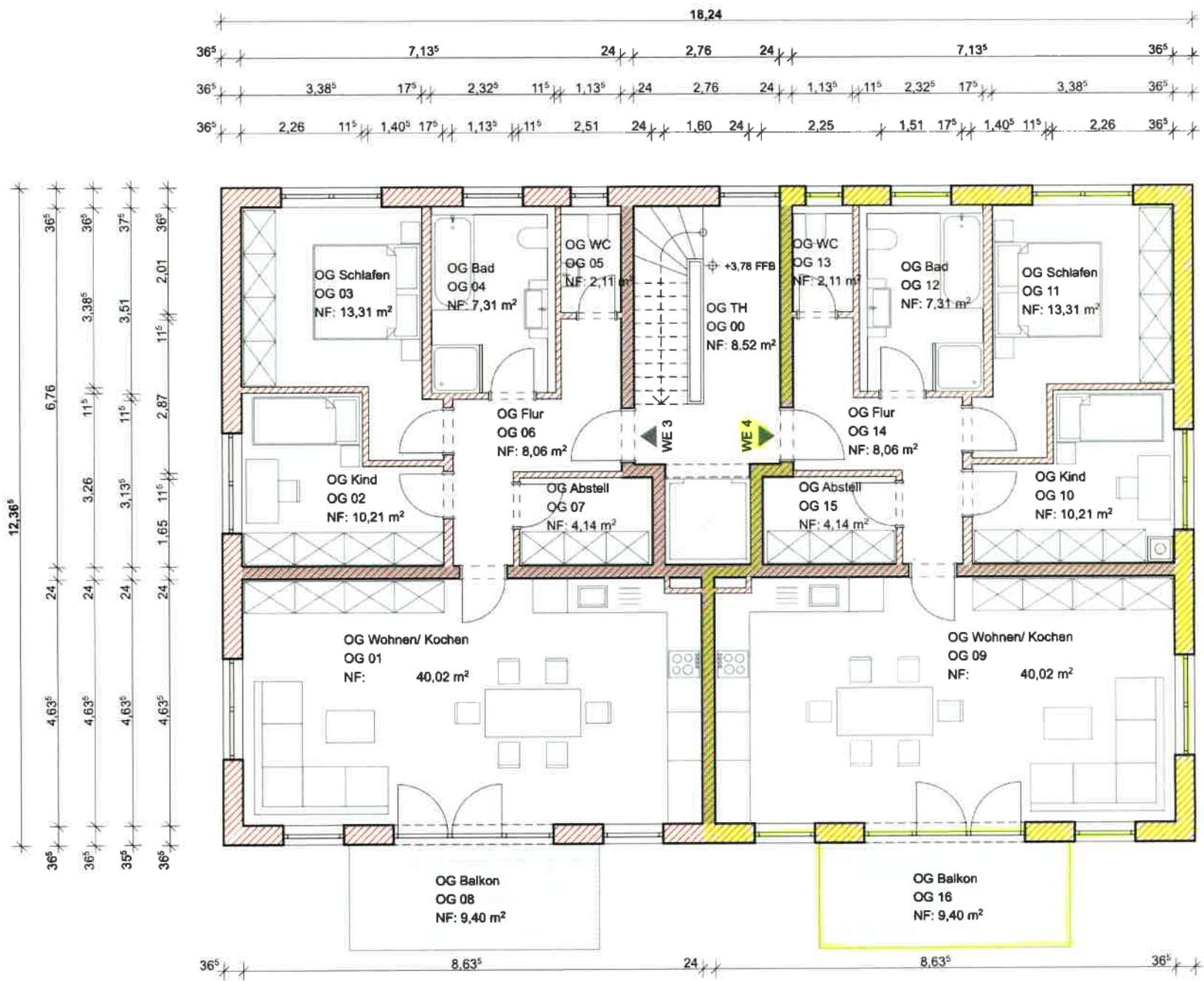
OBERGESCHOß 1:100
